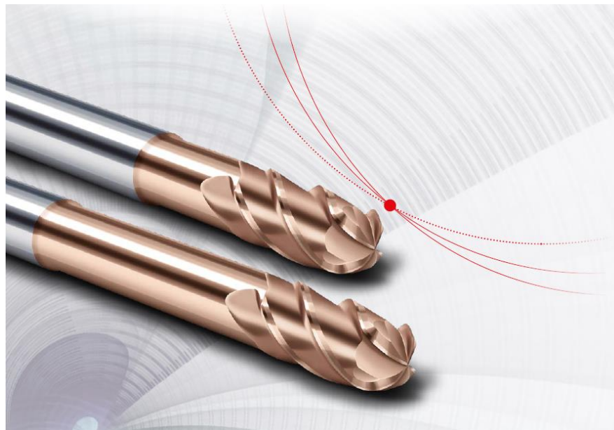
Kulové frézy SpheroX
